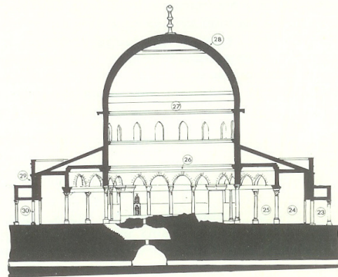
19. ב. כיפת-הסלע. 19. ב. כיפת-הסלע — חתך (ר' איור 1א, 1ב' ותכנית במפה הכללית). מקרא: 23. כניסה; 24. טיילת חיצונית; 25. טיילת פנימית; 26. כתובת מאמון (ר' איור 1א); 27. יציע עם חלונות; 28. כיפת-עץ כפולה, מצופה ברוטנאלומיניום; 29. ציפוי-קיר עליון — חרטינה; 30. ציפוי-קיר
